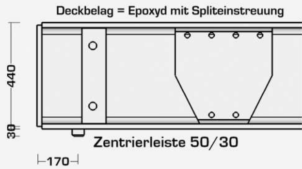
Detail: Auflager
