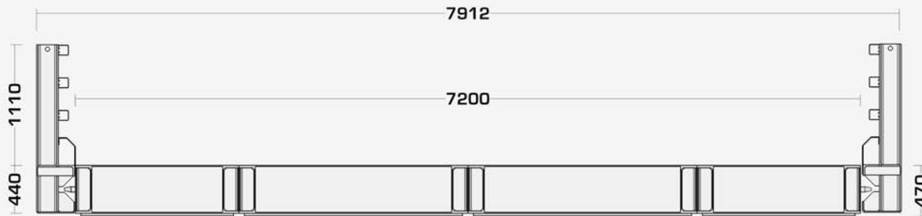
Vorderansicht
