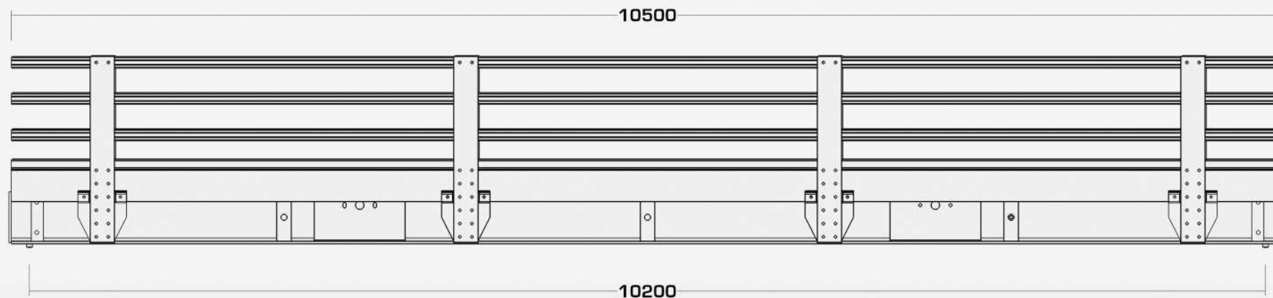
Seitenansicht
