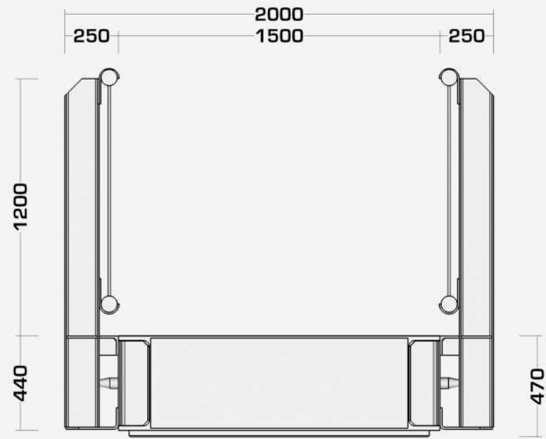
Vorderansicht
