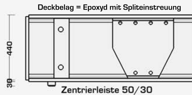
Detail: Auflager
