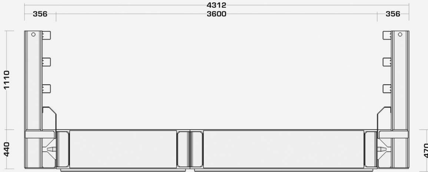
Vorderansicht
