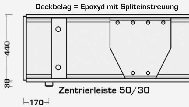
Detail: Auflager
