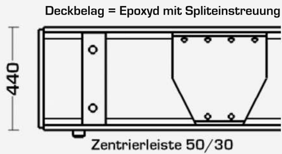
Detail: Auflager
